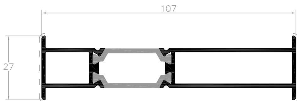
L58862 perfil ligação 107
