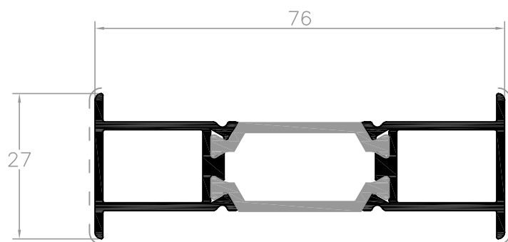
L58861 perfil ligação 76
