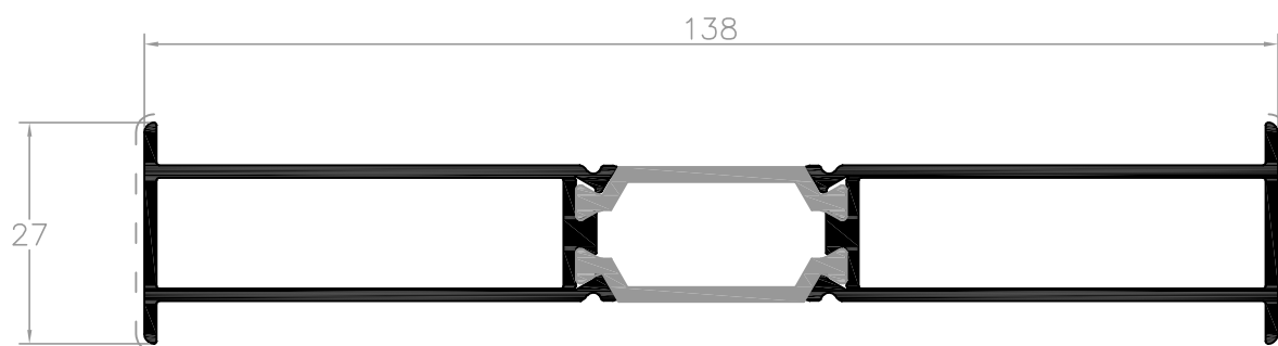
L58863 perfil ligação 139
