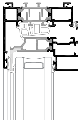
corte vertical escala: 1/2
