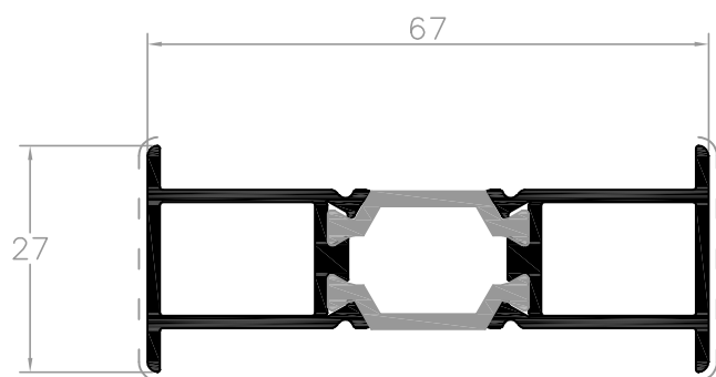
L55861 perfil ligação 67
