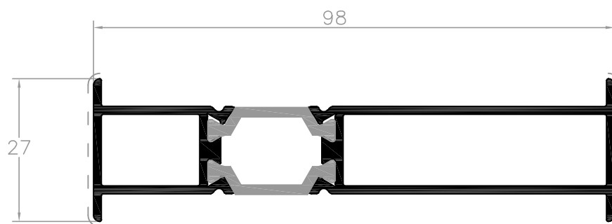
L55862 perfil ligação 98
