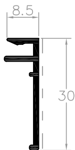
L52761 perfil remate 30 x 8.5
