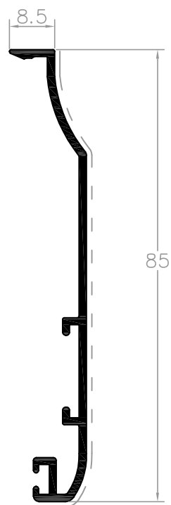
L52765 perfil remate 85 x 8.5
