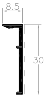
L52762 perfil remate 30 x 8.5
