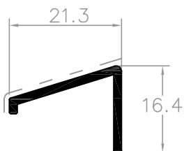
L50804 pingadeira tradicional
