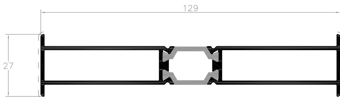
L55863 perfil ligação 129
