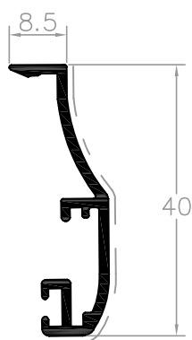
L52763 perfil remate 40 x 8.5
