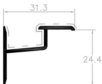
L50813 recolha ressoados
