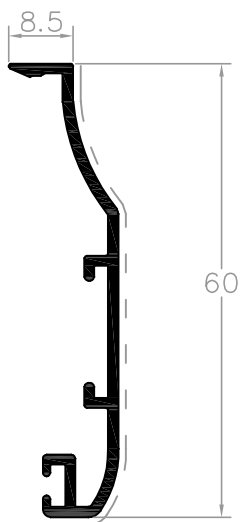
L52764 perfil remate 60 x 8.5
