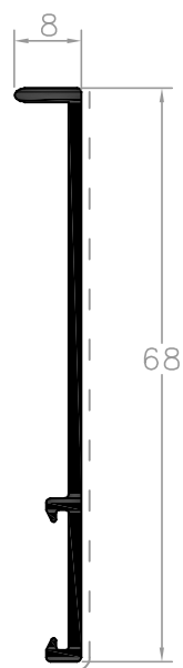
L52766 perfil remate 60 x 8.5
