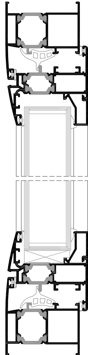
corte vertical escala: 1/2
