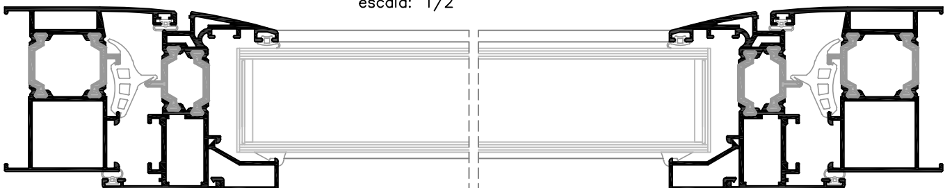
corte horizontal escala: 1/2
